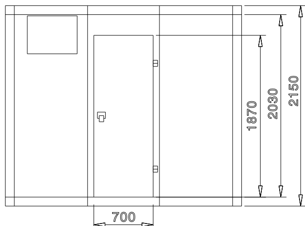
Zij aanzicht
